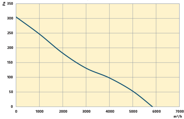
T/AC-A 500-5-25 T4 0,55 kW
