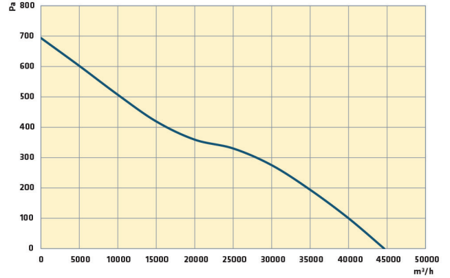
T/AC-A 900-5-40 T4 5,50 kW
