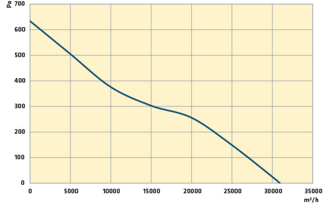
T/AC-A 800-5-35 T4 3,00 kW
