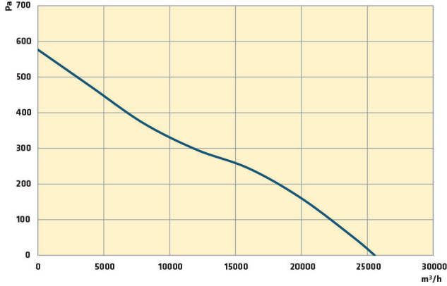
T/AC-A 800-5-30 T4 2,20 kW
