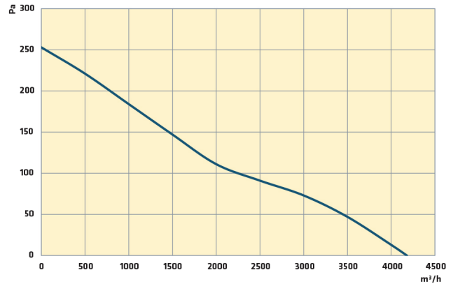
T/AC-A 450-5-25 T4 0,55 kW
