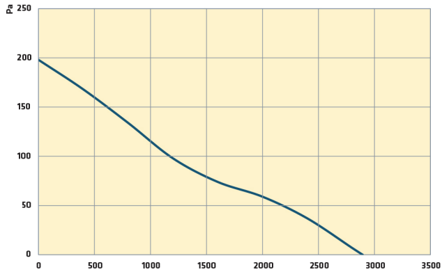
T/AC-A 400-5-25 T4 0,37 kW
