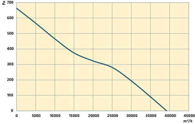
T/AC-A 900-5-35 T4 4,00 kW
