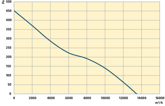
T/AC-A 630-5-30 T4 1,10 kW
