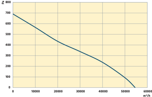
T/AC-A 1000-5-40 T4 7,50 kW
