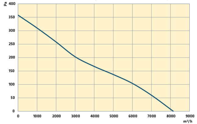
T/AC-A 560-5-25 T4 0,75 kW
