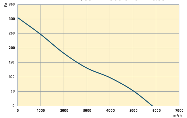
T/CC-ATX 500-5-25 T4 0,55 kW
