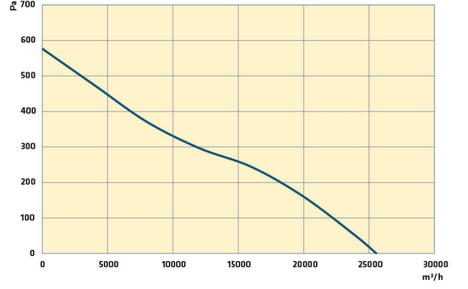
T/CC-ATX 800-5-30 T4 2,20 kW
