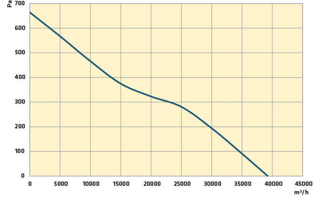
T/CC-ATX 900-5-35 T4 4,00 kW
